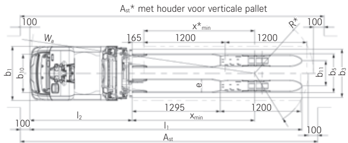
Bovenaanzicht OPX-L 16
