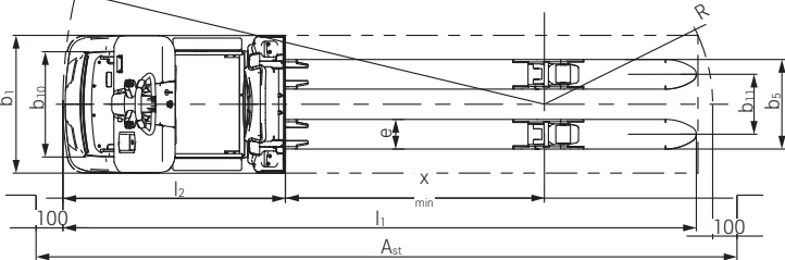
Bovenaanzicht OPX 20/25/OPX 20 Plus/OPX 25 Plus
