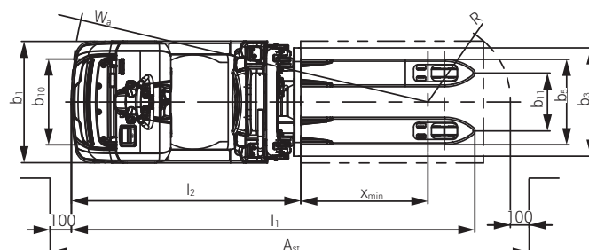
Bovenaanzicht OPX-D 20
