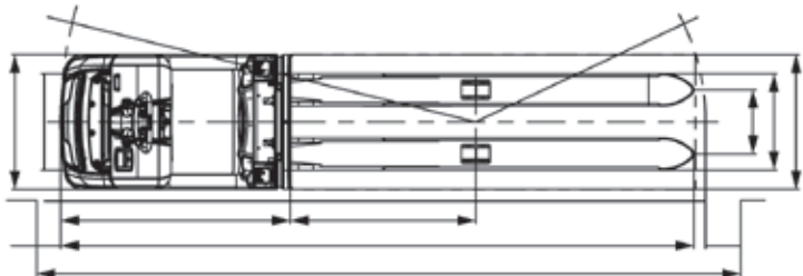
Bovenaanzicht OPX-L 16
