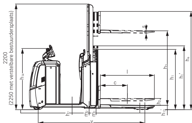
Zijaanzicht OPX-D 20
