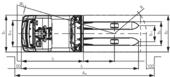
Bovenaanzicht OPX-L 12
