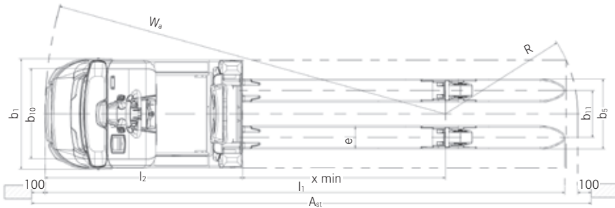
Bovenaanzicht OPX 20 iGo neo
