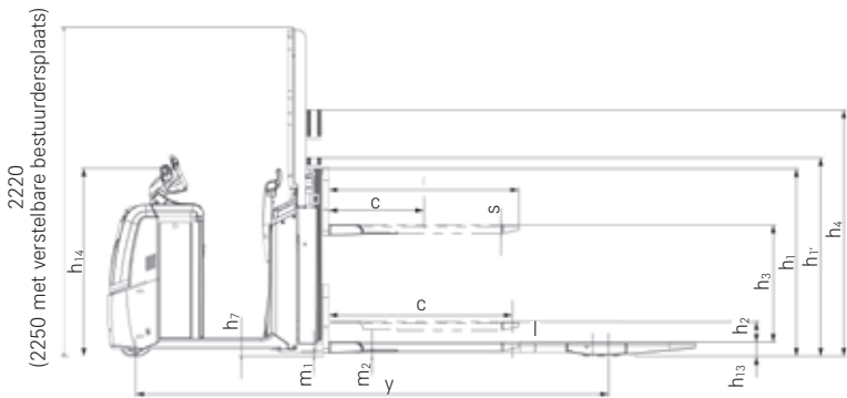
Zijaanzicht OPX-L 20
