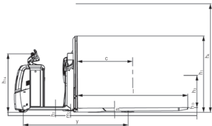
Zijaanzicht OPX-L 16
