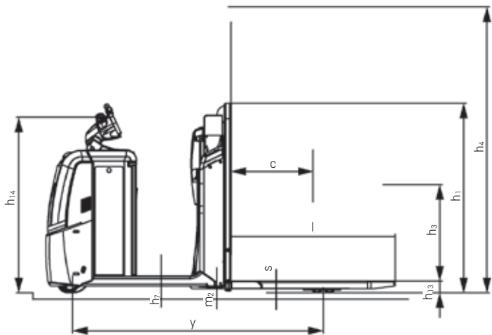
Zijaanzicht OPX-L 12
